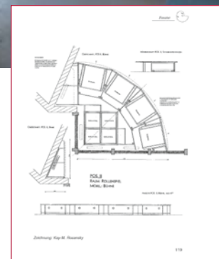
Abb. 4–6: Ein Podest (für das Rollenspiel) entsteht: Entwurf – technische Zeichnung – Fertigstellung in Schreinerarbeit
